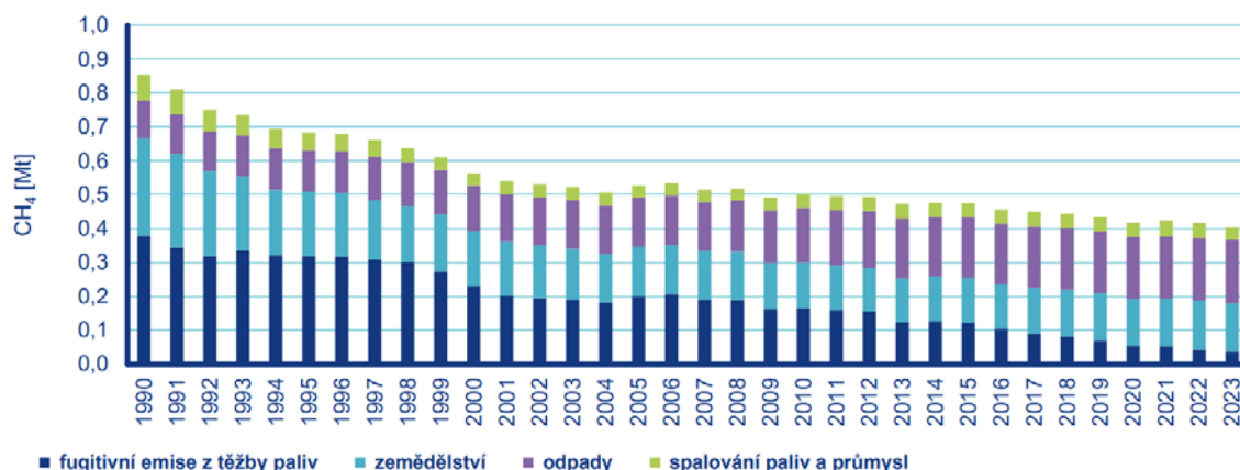
Obrázek 20 Podíl jednotlivých sektorů na emisích \text{CH}_4 , 1990–2023 (ČHMÚ, 2024)
