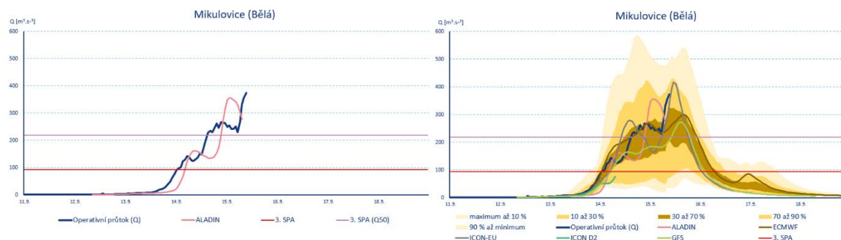
Obr. 3.2.4 Pozorovaný průtok (modrá čára) a předpověď pro Bělu v Mikulovicích z 12. září 07:00 ve verzi pro veřejnost – HPPS (jedna varianta) a v pravděpodobnostní verzi, se kterou pracuje předpovědní služba.
