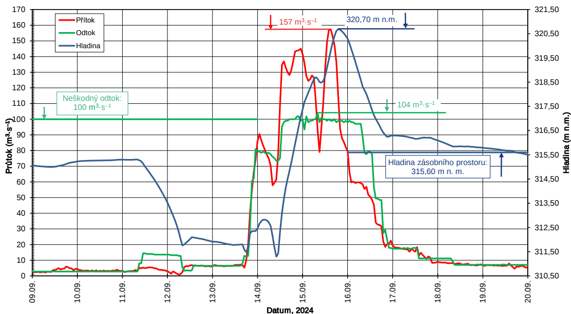
VD Les Království – povodeň září 2024 Časový průběh přítoku vody do nádrže, odtoku z nádrže a hladiny v nádrži
