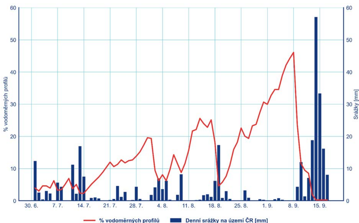
Obr. 2.1.1 Vývoj hydrologického sucha ve vodoměrných stanicích v letních měsících až do srážkové situace v září.
