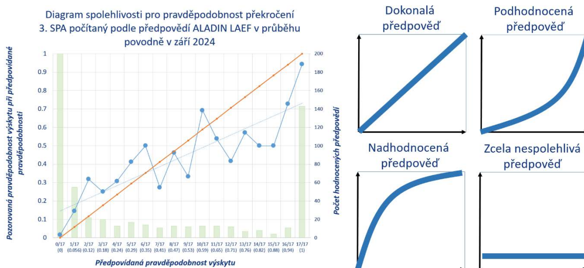
Obr. 3.2.5. Diagram spolehlivosti pro hydrologické pravděpodobnostní předpovědi počítané podle 17 variant srážek z meteorologického předpovědního systému ALADIN LAEF. Souhrnné výsledky pro všechny předpovědní stanice za září 2024. V pravé části vysvětlení pro čtení diagramu.
