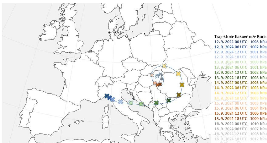
Obr. 1.1.7 Trajektorie tlakové níže Boris při zemi od 12. 9. 22 UTC do 16. 9. 18 UTC.
