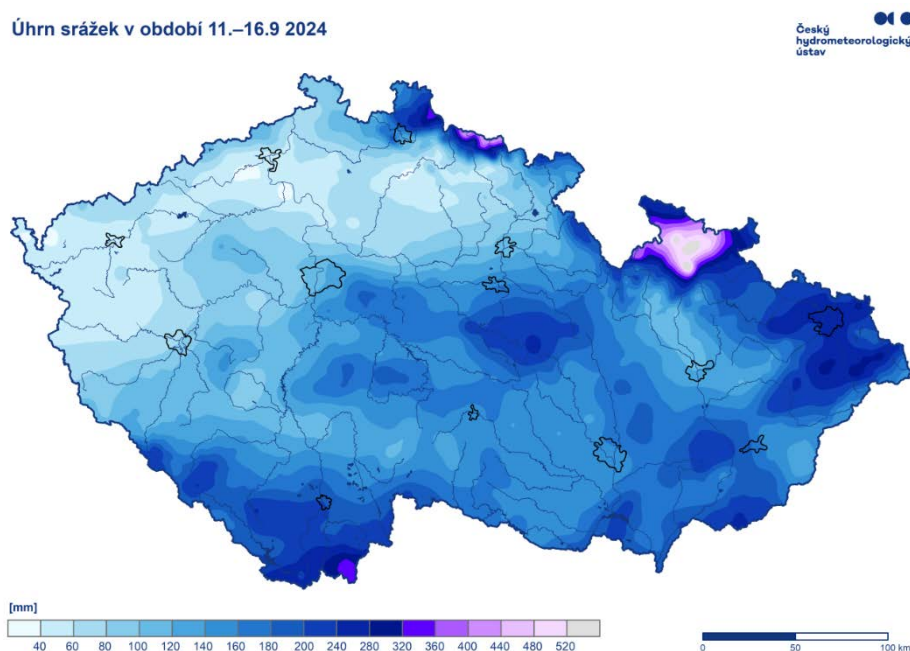
Obr. 1.3.2 Šestidenní úhrn srážek v období 11.–16. 9. 2024.
