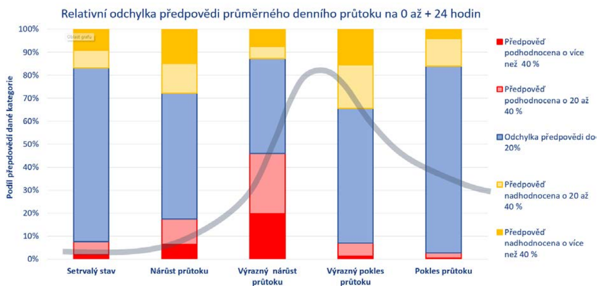
Obr. 3.2.6 Odchylky předpovědi průtoků ve smyslu nadhodnocení nebo podhodnocení pozorovaného průtoků v závislosti na odtokové fázi v průběhu povodně.
