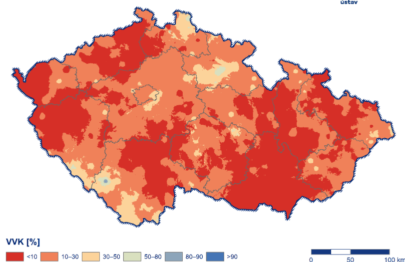
Obr. 1.1.4 Balance vody v půdě vyjádřená v % využitelné vodní kapacity půdy ke dni 9. 9. 2024.
